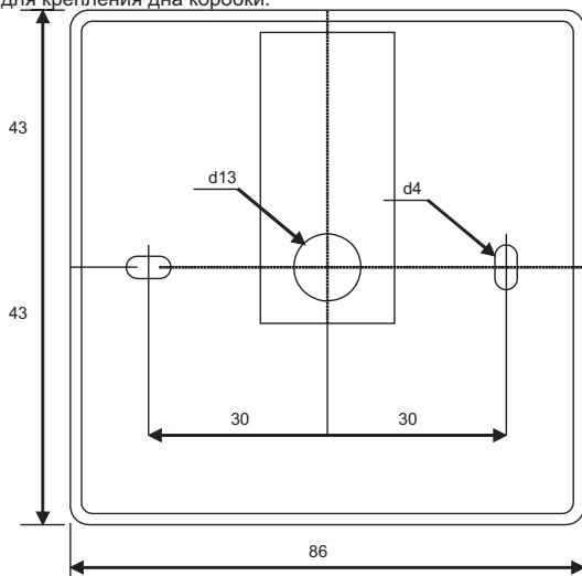
Чертеж крепления
